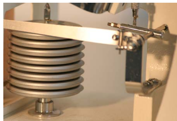
Druckmessdose
