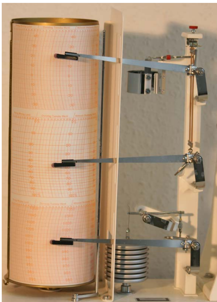
Klimamessgerät
